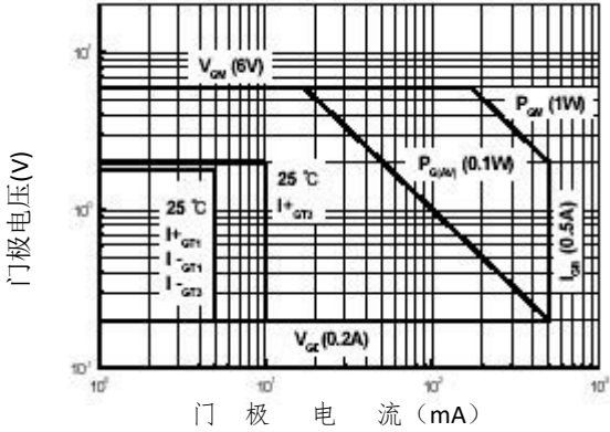
图一、门极特性
