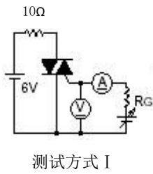
图九、门极触发特性测试电路
