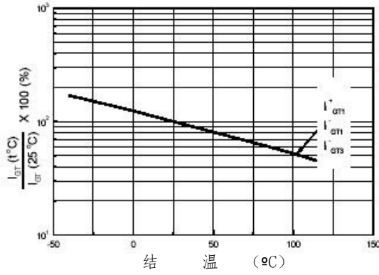
图七、门极触发电流——结温
