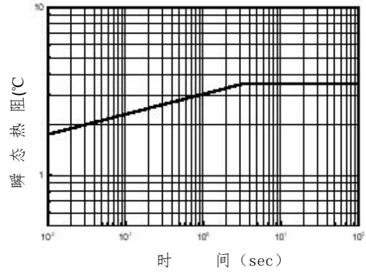
图八、瞬态热阻
