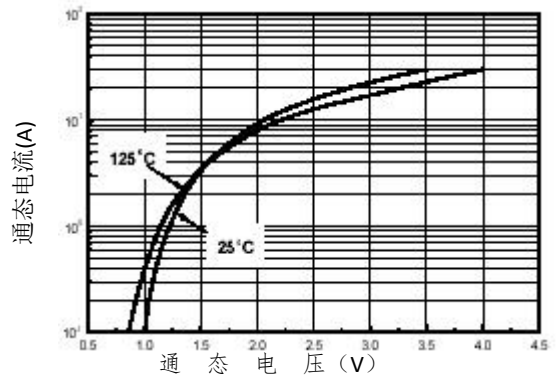
图二、通态电压
