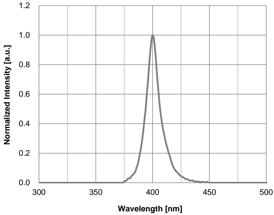
Fig 1. Spectrum, T_s=25^\circ\text{C} , I_F=180\text{mA}
