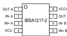
图4.3 SOIC8封装
