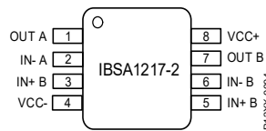
图4.4 MSOP8封装
