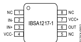
图4.2 MSOP8封装
