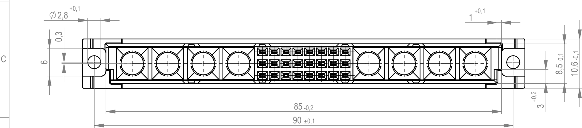
Bestückungsplan / contact layout
