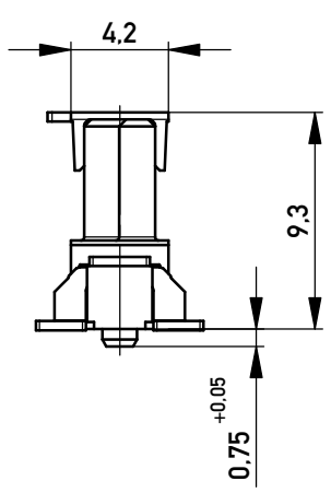
ohne Ansaughaube - without hood
