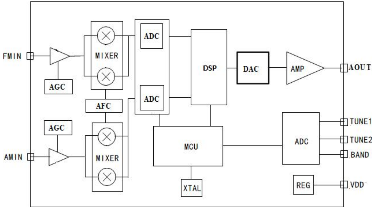
FSV4825-A10 内部功能框图
