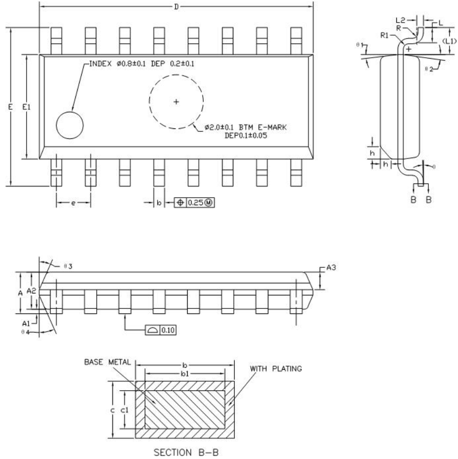
封装尺寸图:
