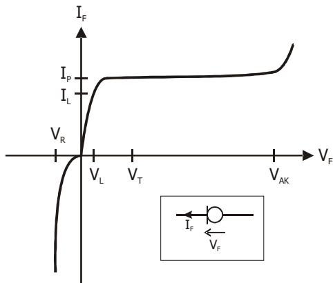
Fig. 1 Characteristic and symbol Kennlinie und Symbol
