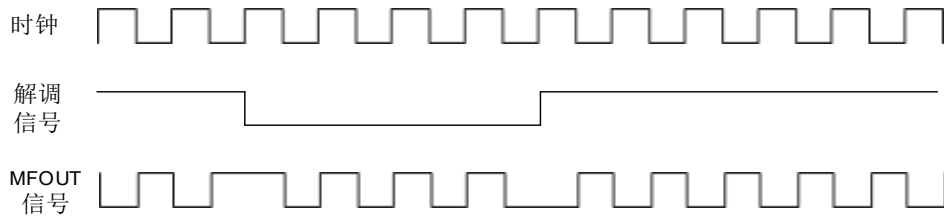
图 10.5 SAM 模式 MFIN 信号波形示意图
