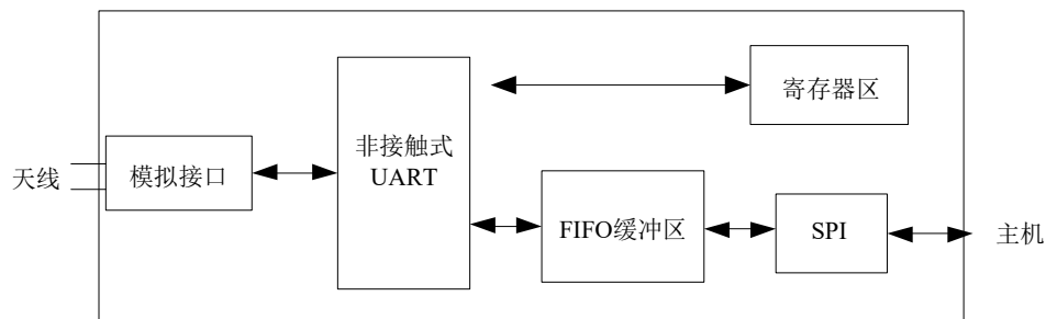
图 5.1 Ci523 简化框图
