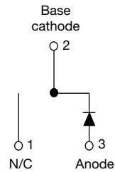
VS-8ETU04SHM3
