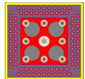
Figure 9 : Top Layer + Top Paste
