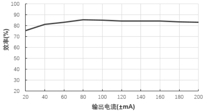
效率Vs输出电流(Vin=12V)@A1205S-2WR3
