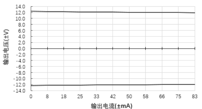
输出电压Vs输出电流(Vin=24V)@A2412S-2WR3
