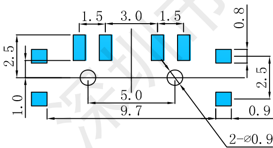
P. C. B. Land Pattern
