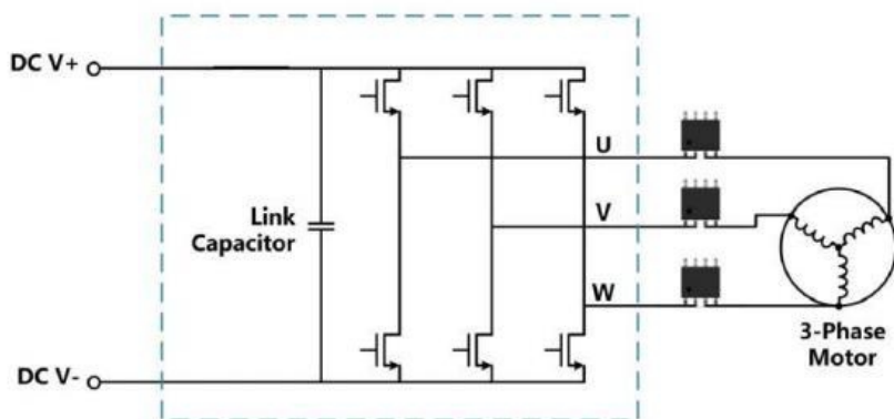
3 相电机控制应用电路
