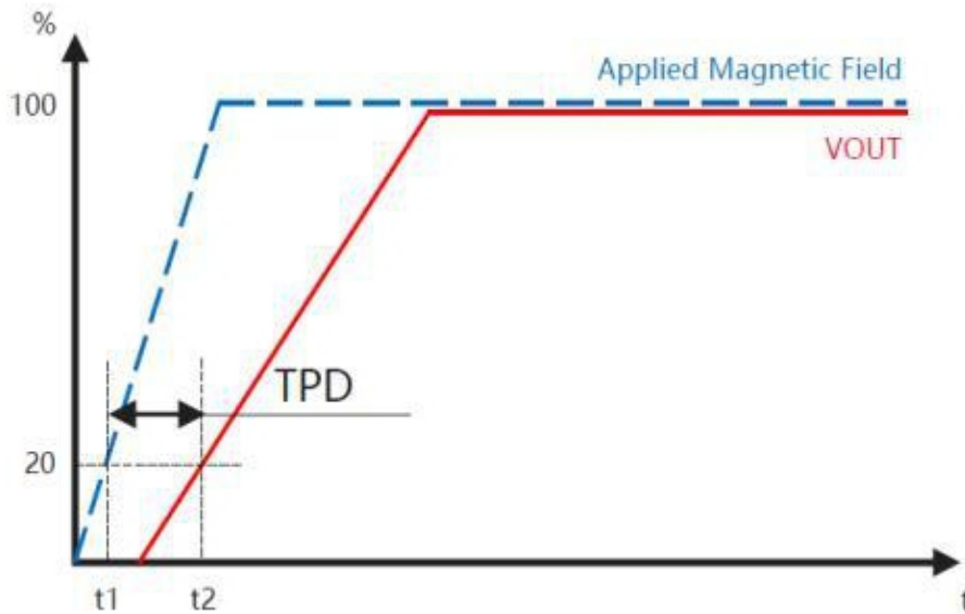
图 2：传输延迟定义
