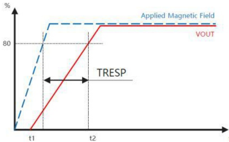
图 4：响应时间定义
