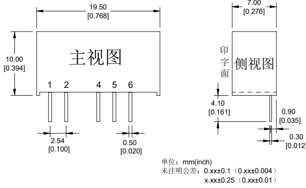
封装尺寸图
