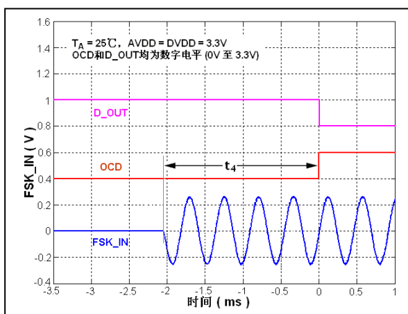
图 13. 载波检测开启时序
