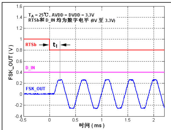
图 11. 载波起始时间
