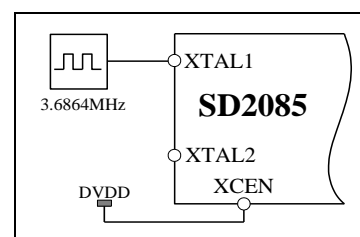
图9. 外灌CMOS时钟连接
