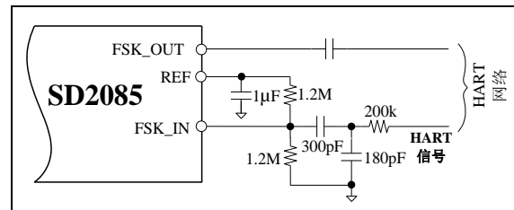
图6. SD2085 外部带通滤波器连接
