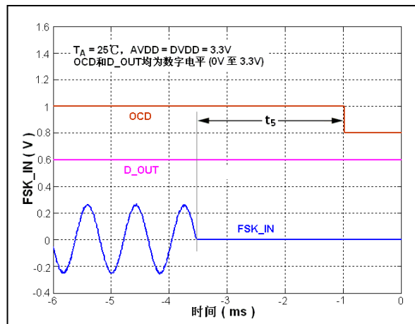
图 14. 载波检测关闭时序
