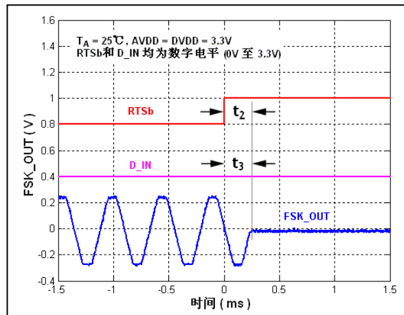
图 12. 载波停止/衰减时间
