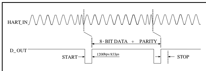
图7. SD2085 解调波形图
