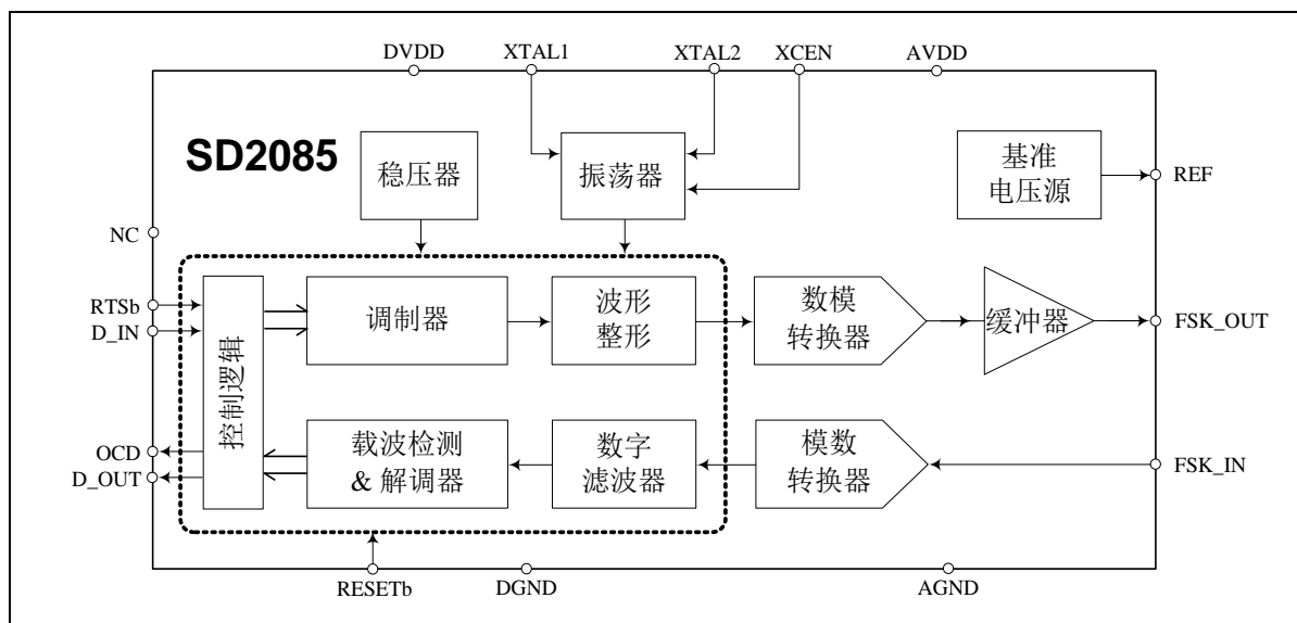
图 2. 功能框图
