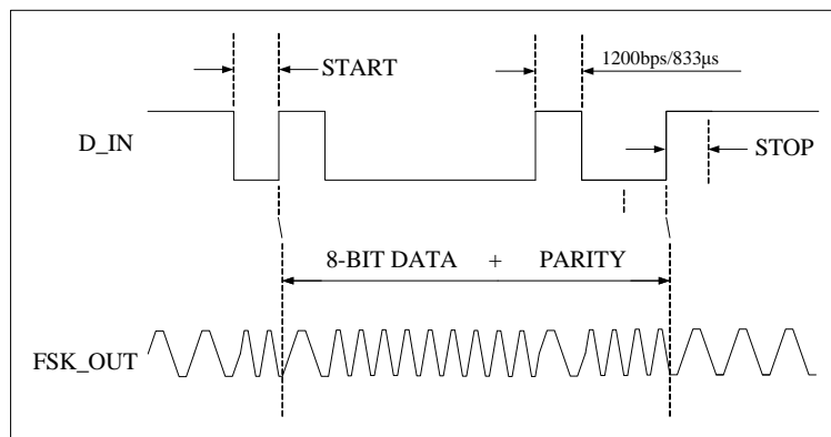
图4. SD2085 调制波形图
