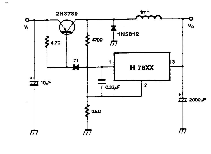
图13、开关稳压器
