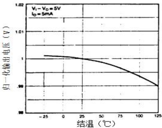
输出电压
