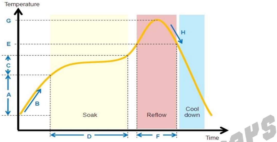
图 10-1 AXP313A 典型回流焊曲线
