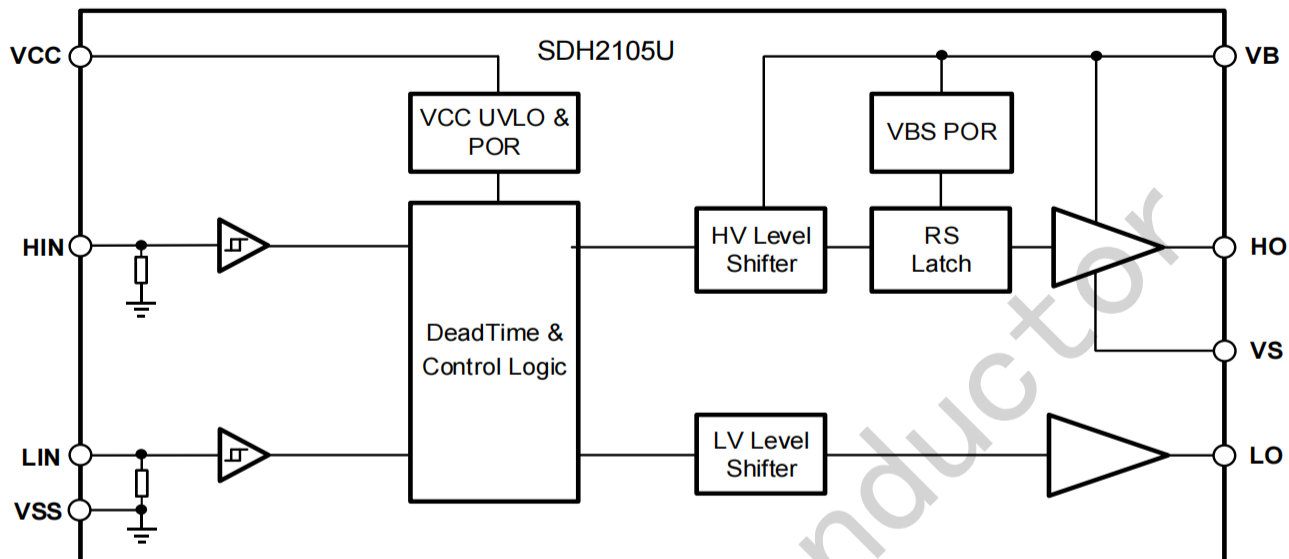
图7-1 SDH2105U的功能框图
