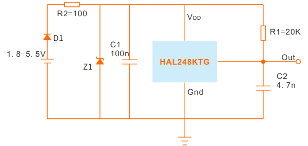
反向保护应用电路
