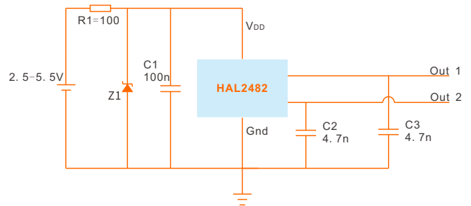
反向保护应用电路
