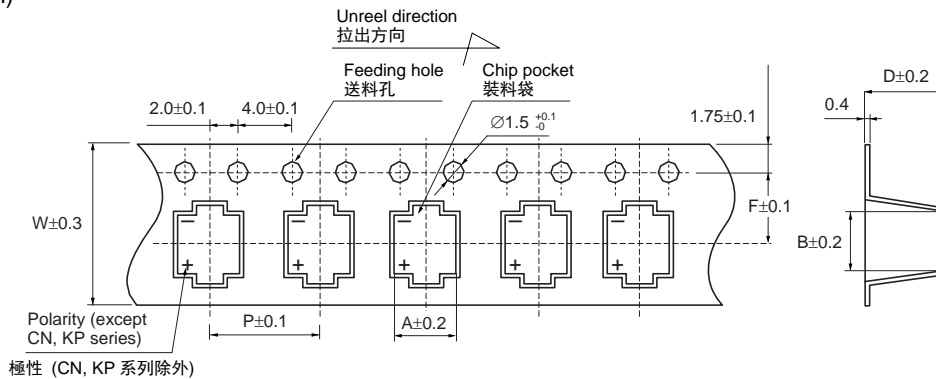
Dimension 尺寸表 (Unit: mm)
