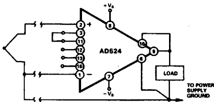
b. Thermocouple
