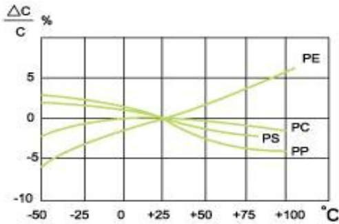
容量变化率与温度的关系
