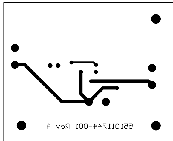
Bottom Layer
