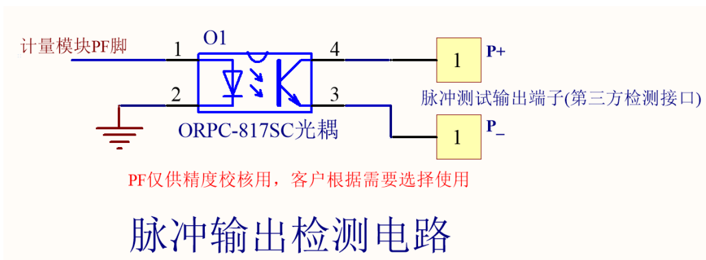
IM1281C 脉冲检测接口接线示意图
