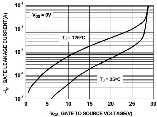
Figure 12. I_{gss} vs. V_{gss}
