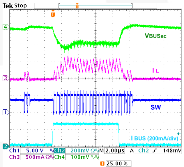
Figure 32. Load Transient, 5\text{-}255\text{-}5\text{ mA} , t_R=t_F=100\text{ ns}
