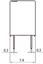
Dimensions尺寸
