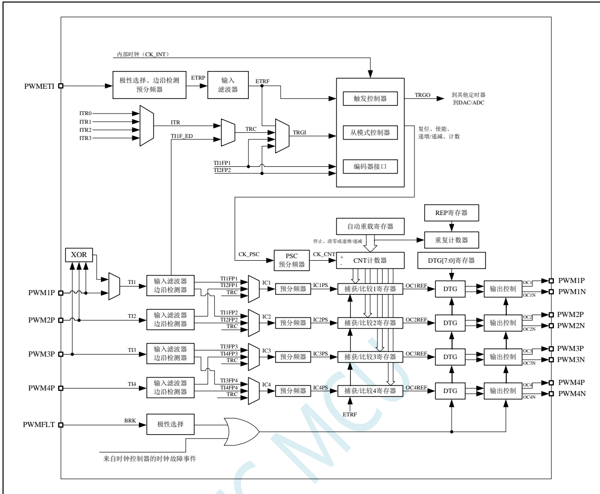
高级 PWM 定时器内部结构框图
