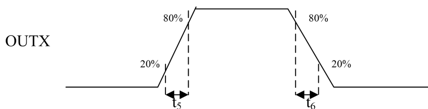
图 3 GC9111 输入输出时间参数 2
