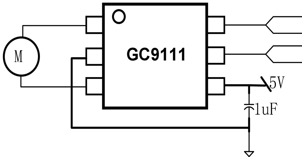
图 4 GC9111 典型应用原理图
