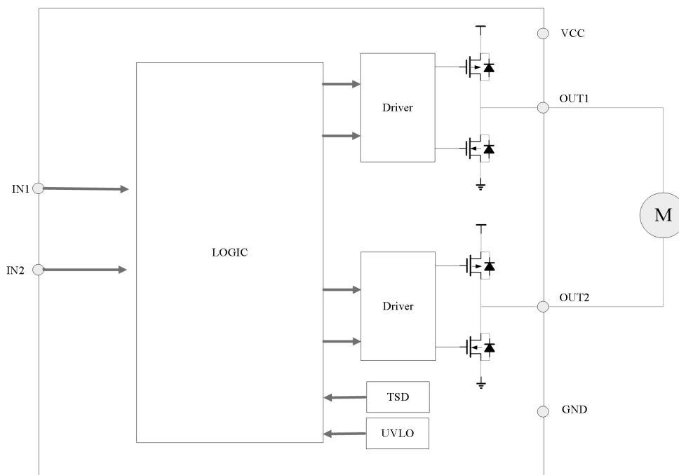
图 1 GC9111 内部框图
