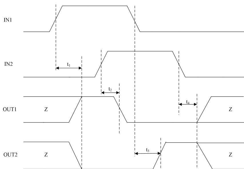
图 2 GC9111 输入输出时间参数 1
