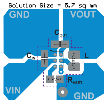
图 9-29. Layout Example
