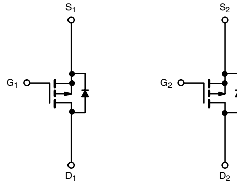
P-Channel MOSFET
