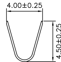
SEC:A-A
