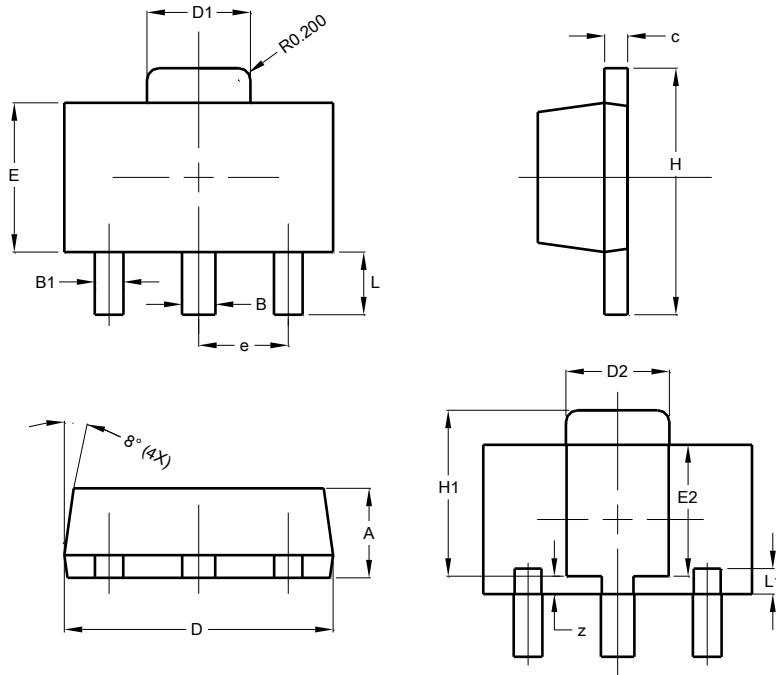
SOT89
