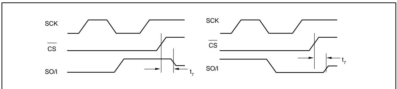
图 11. 高阻输出时序图
