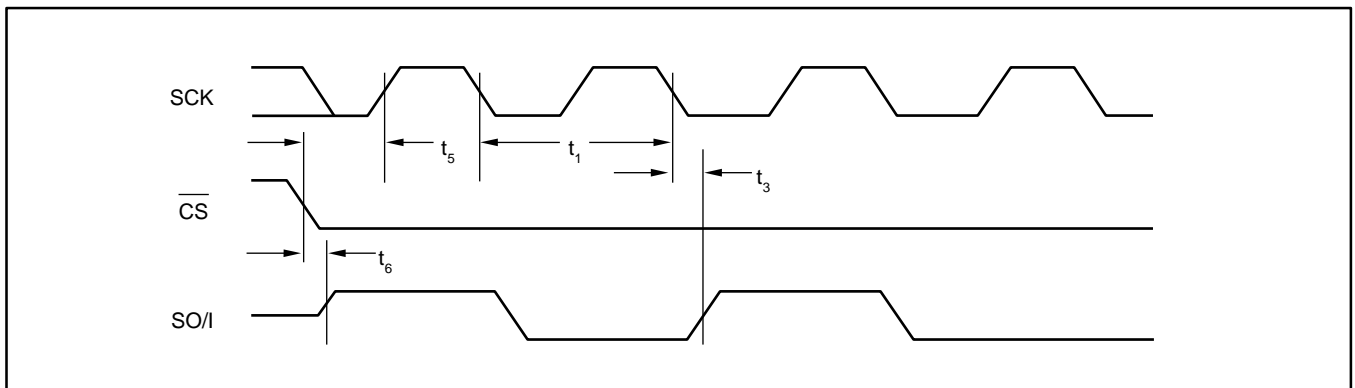
图 10. 输出数据时序图.
