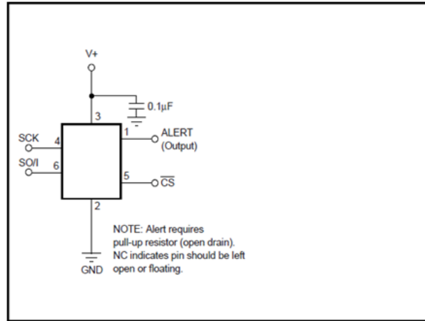
图 1. GX122 典型连接
