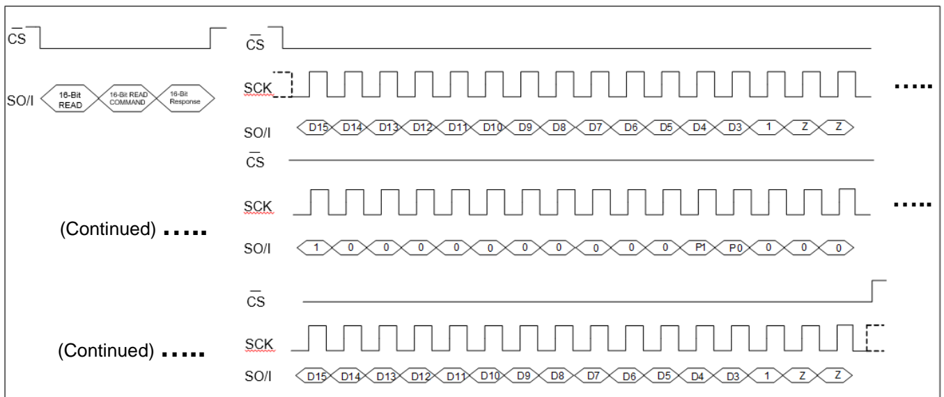
图 5. 读然后发送读命令并读取结果.
