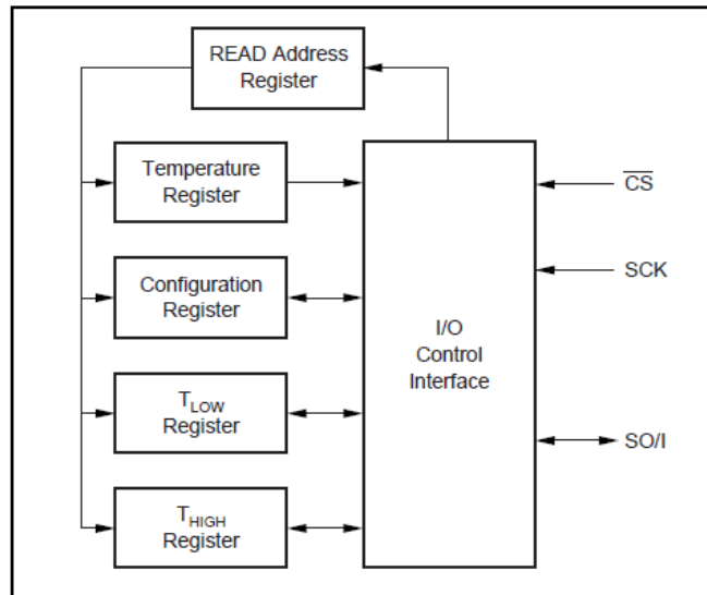
图 7. GX122 的内部寄存器结构
