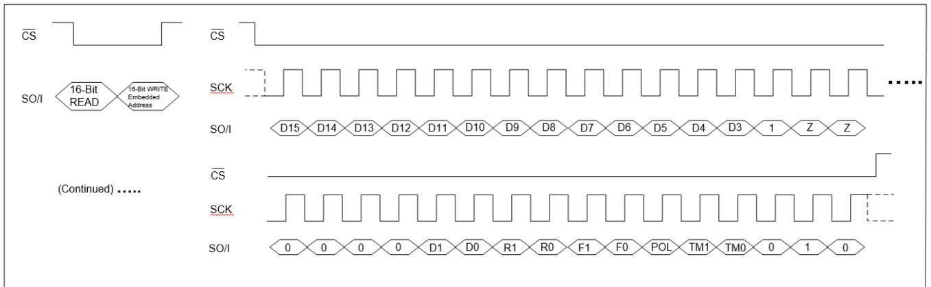
图 4. 读写控制寄存器
