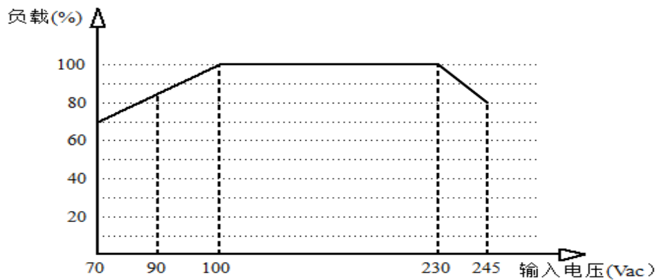
输入电压与负载特性曲线
