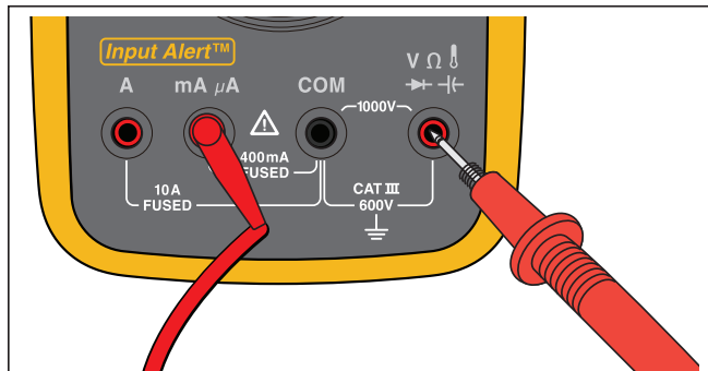
图 7. 测试保险丝
