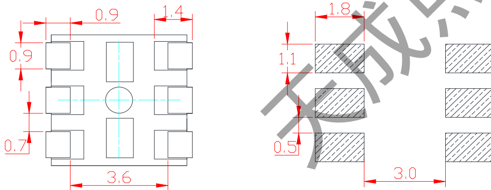
建议焊盘尺寸
