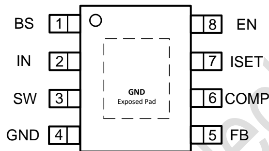
ESOP8
