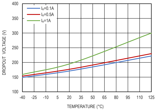
图 12. 压差电压和负载电流的关系, V_{OUT}=3.0V
