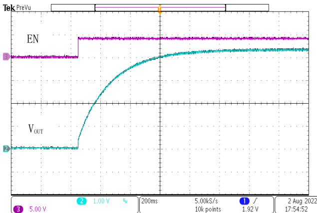
图 20. 软启动, V_{IN}=4.3V , V_{OUT}=3.3V , I_{OUT}=1A
