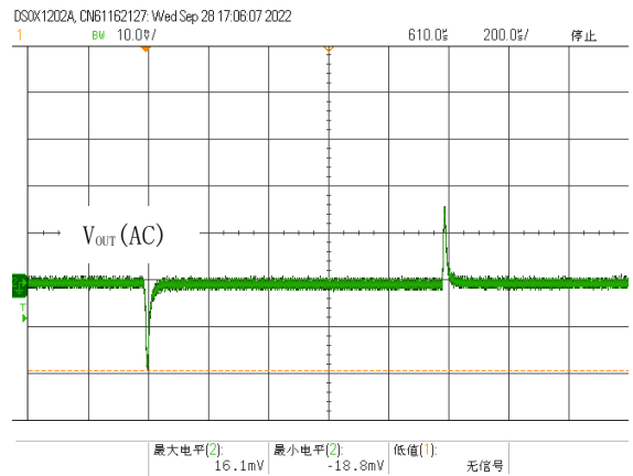
图 21. 负载瞬态响应, V_{IN}=4.3V , V_{OUT}=3.3V , I_{OUT}=1mA to 1A
