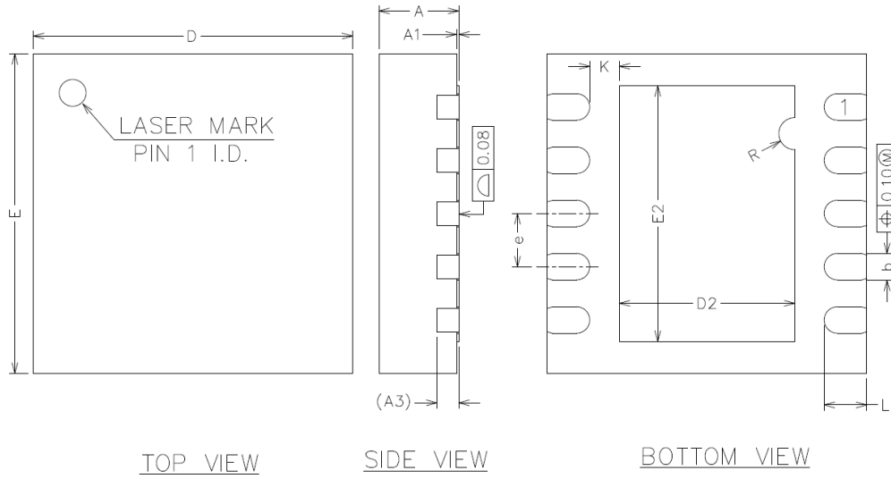
图 24. DFN 封装 (3mmx3mm)
