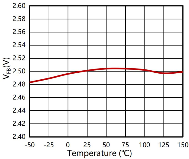
图 11、EA 输入基准电压 V FB 随温度变化曲线
