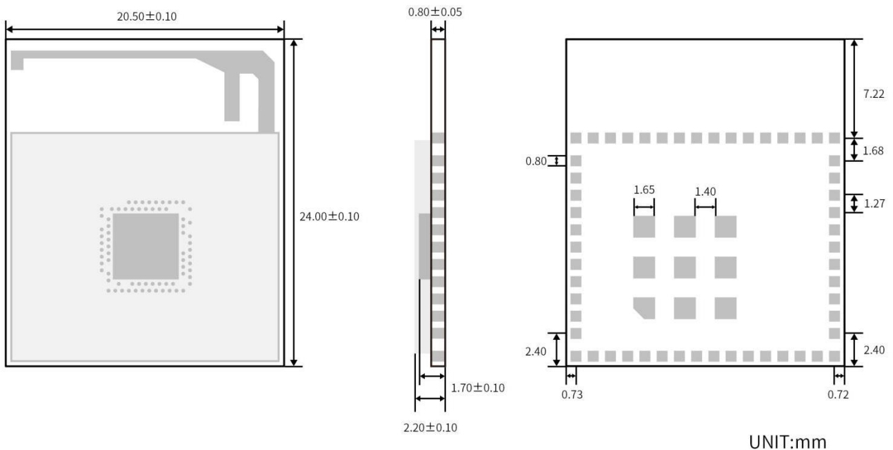
图 2. RF-BM-ND06 尺寸图
