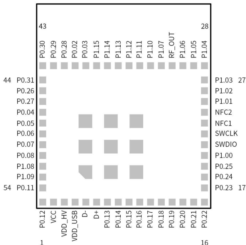
图 3. RF-BM-ND06 引脚图
