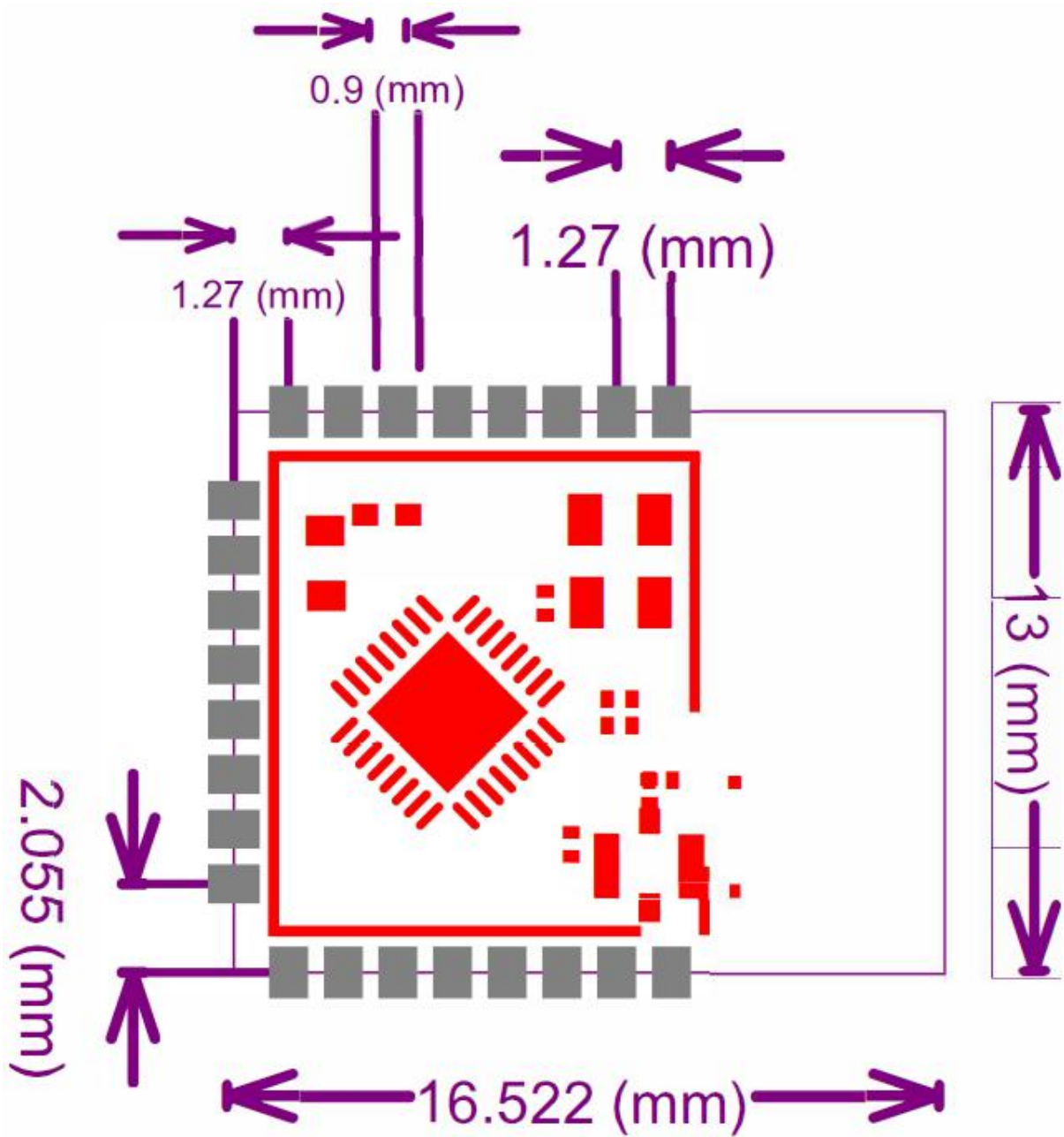
图 1 芯片尺寸图
