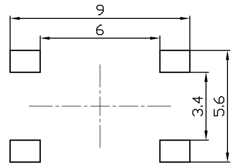
安装参考图
