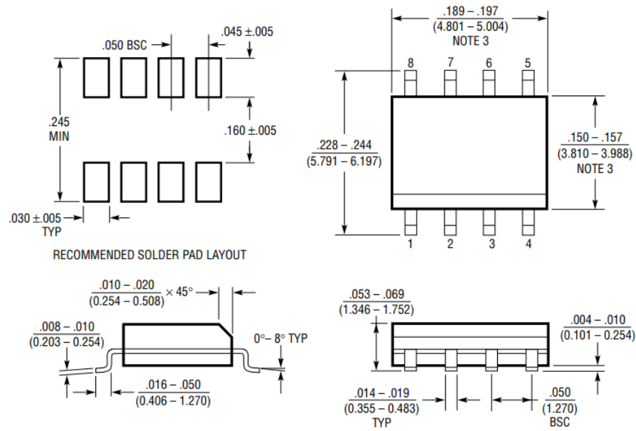
图 23. 8 引脚 SOP-8
