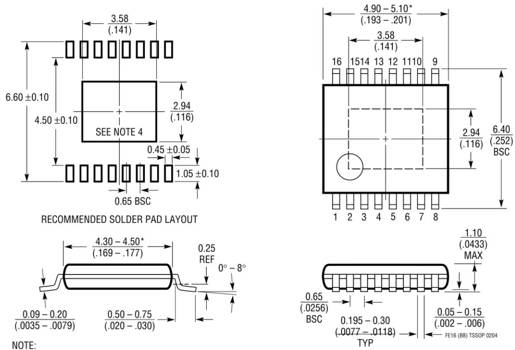
图 24. 16 引脚 TSSOP
