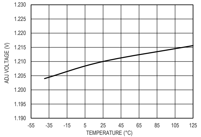
图 12. ADJ 引脚电压精度
