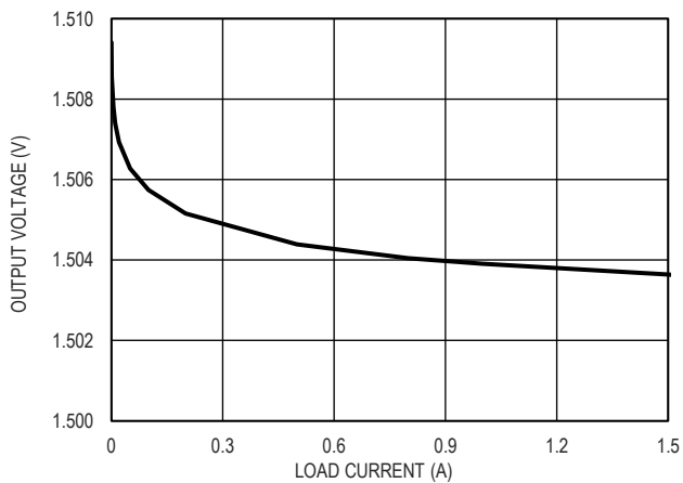
图 9. 1.5V 输出电压和负载电流的关系
