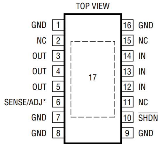
16 引脚 TSSOP 裸露焊盘必须焊接到 PCB 上 图 4 引脚配置
