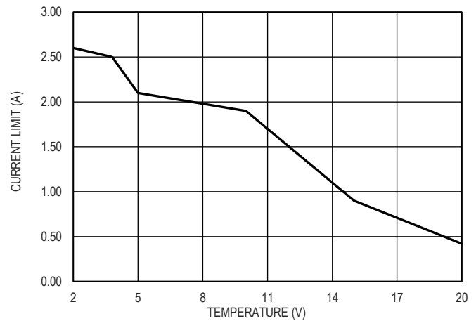
图 14. 输出限流值和输入输出压差的关系
