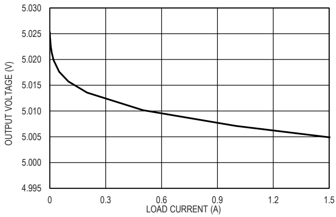
图 11. 5.0V 输出电压和负载电流的关系
