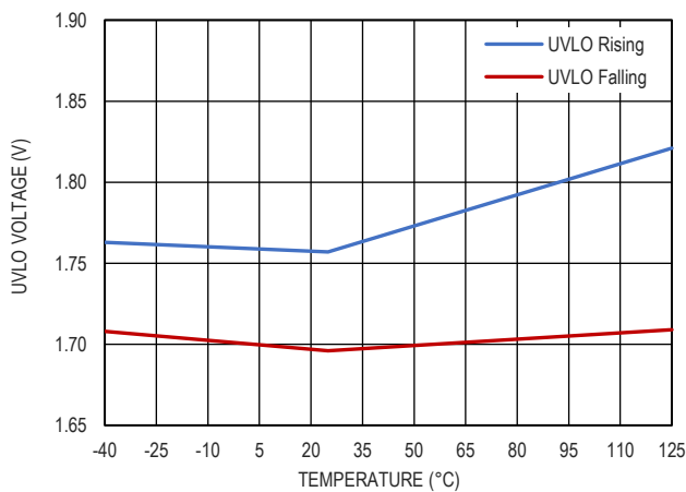
图 15. UVLO 阈值
