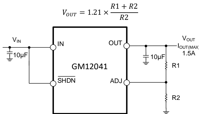
图 21. 由外部电阻决定的输出电压
