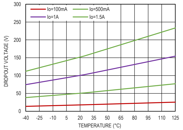
图 6. 压差电压和温度的关系
