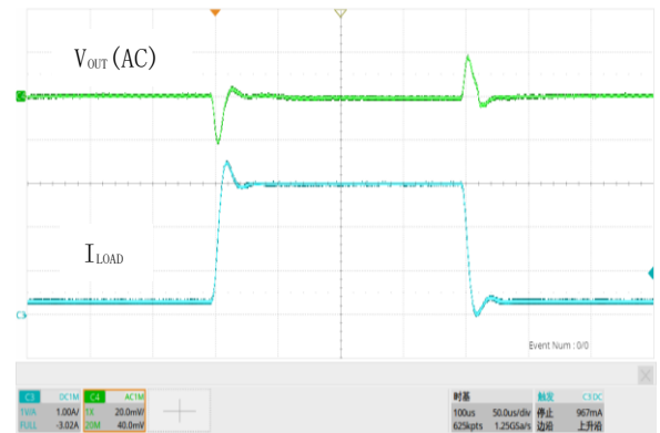
图 20. 负载瞬态响应, V_{IN}=2.8V , V_{OUT}=1.8V , I_{OUT}=0.1A to 1.5A
