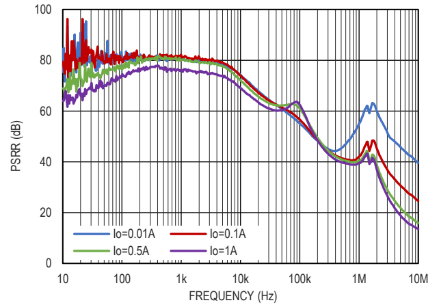
图 18. 电源电压纹波抑制比, V_{IN}=5V , V_{OUT}=3.3V
