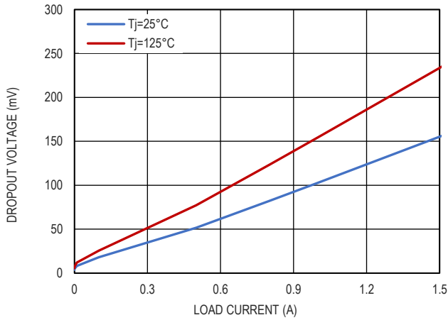
图 5. 压差电压和负载电流的关系
