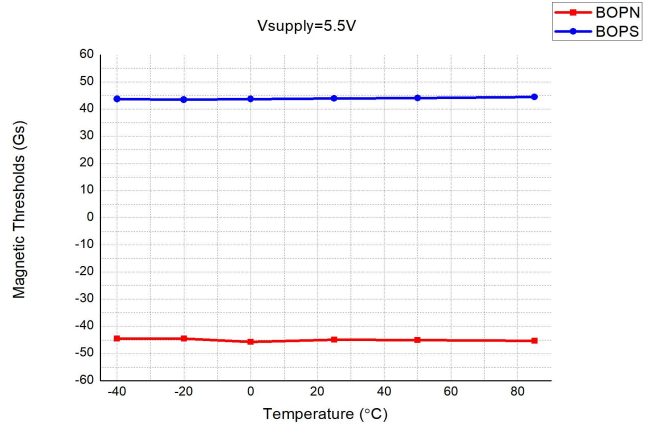
磁场阈值 vs 温度 @VDD=5.5V
