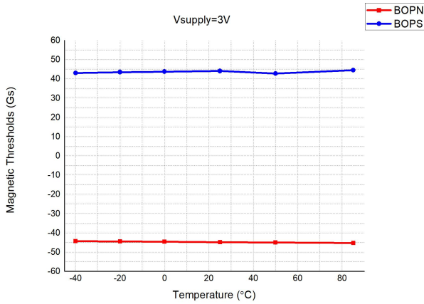
磁场阈值 vs 温度 @VDD=3.0V
