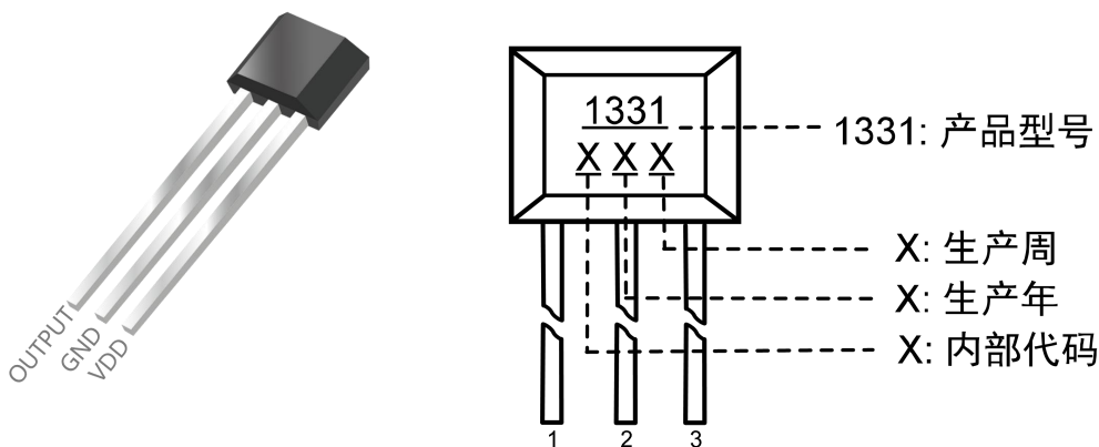
引脚结构 (俯视图)
