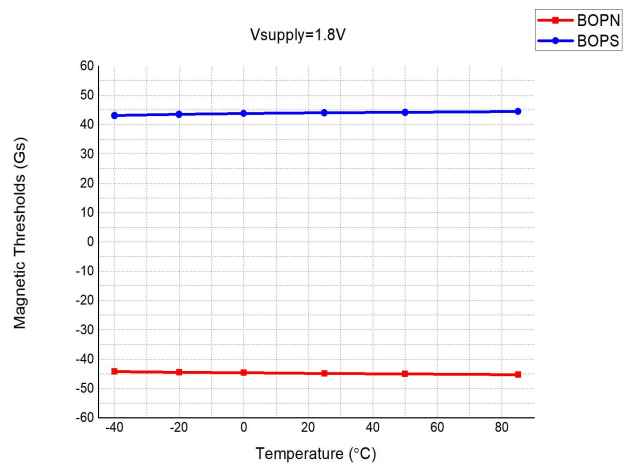
磁场阈值 vs 温度 @VDD=1.8V
