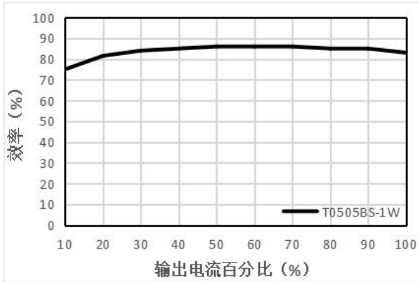
效率VS输出负载 (Vin=5V)
