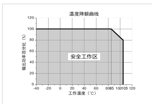
输出功率与工作温度关系曲线图
