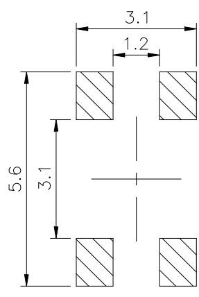
PCB. 焊接图
